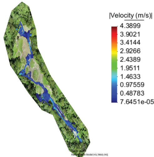
Figura 3. Velocidad con hidrograma T 50 +18%, sitio arqueológico.
