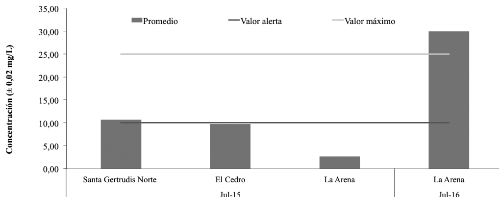
Figura 5. Concentraciones de fosfatos obtenidas en los acueductos ASADA del cantón de Grecia.
