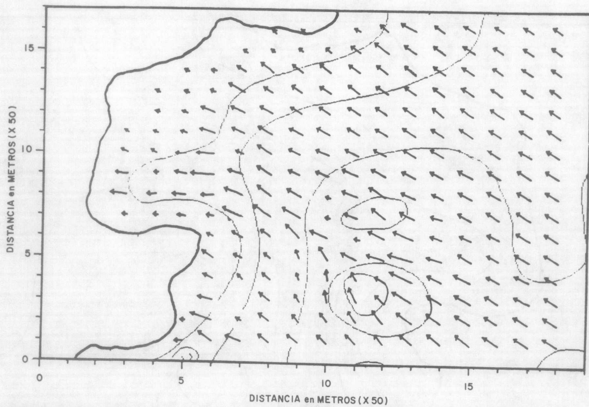
FIGURA 6-a. Vectores de ola en Playa Carbón, provincia de Guanacaste, para H_s=1,2 m, T=4,5 s y O_s=5,2 grd.
