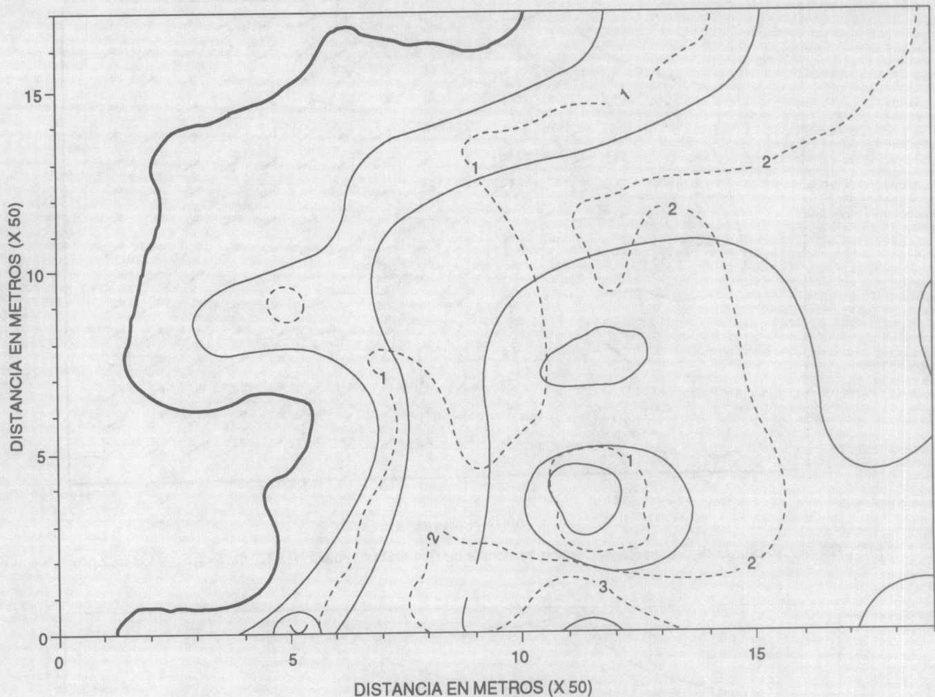
FIGURA 7. Contornos de altura de ola (m) en Playa Carbón, Guanacaste, para H_s=4,9 m, T=14,5 s y O_s=22 grd.
