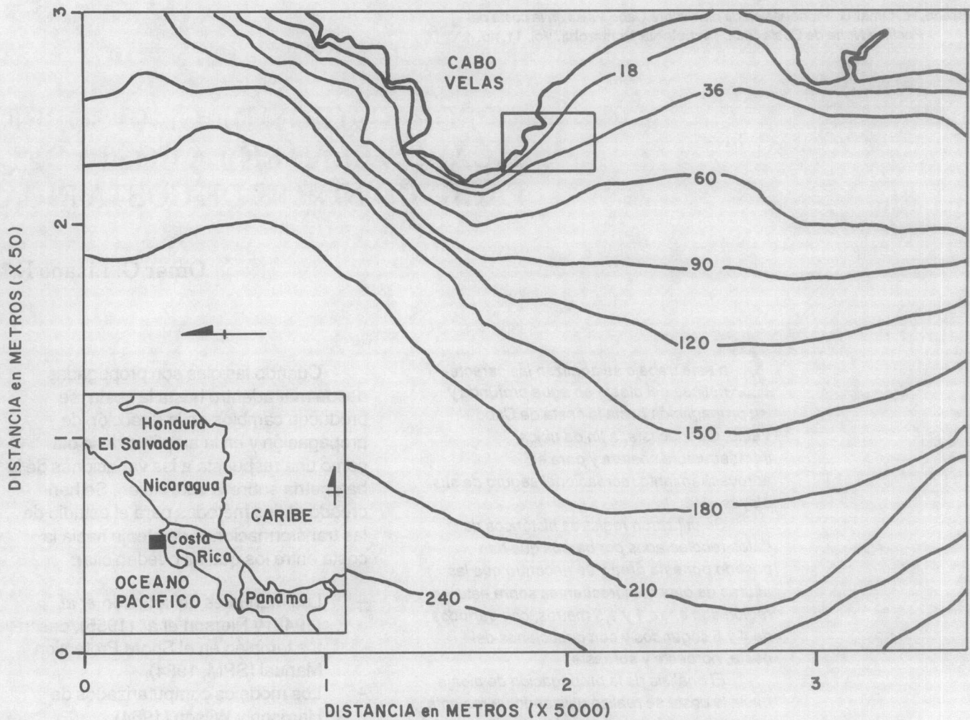
FIGURA 1. Contornos batimétricos (pies) frente a Cabo Velas, provincia de Guanacaste (1 m = 3,28 pies).
