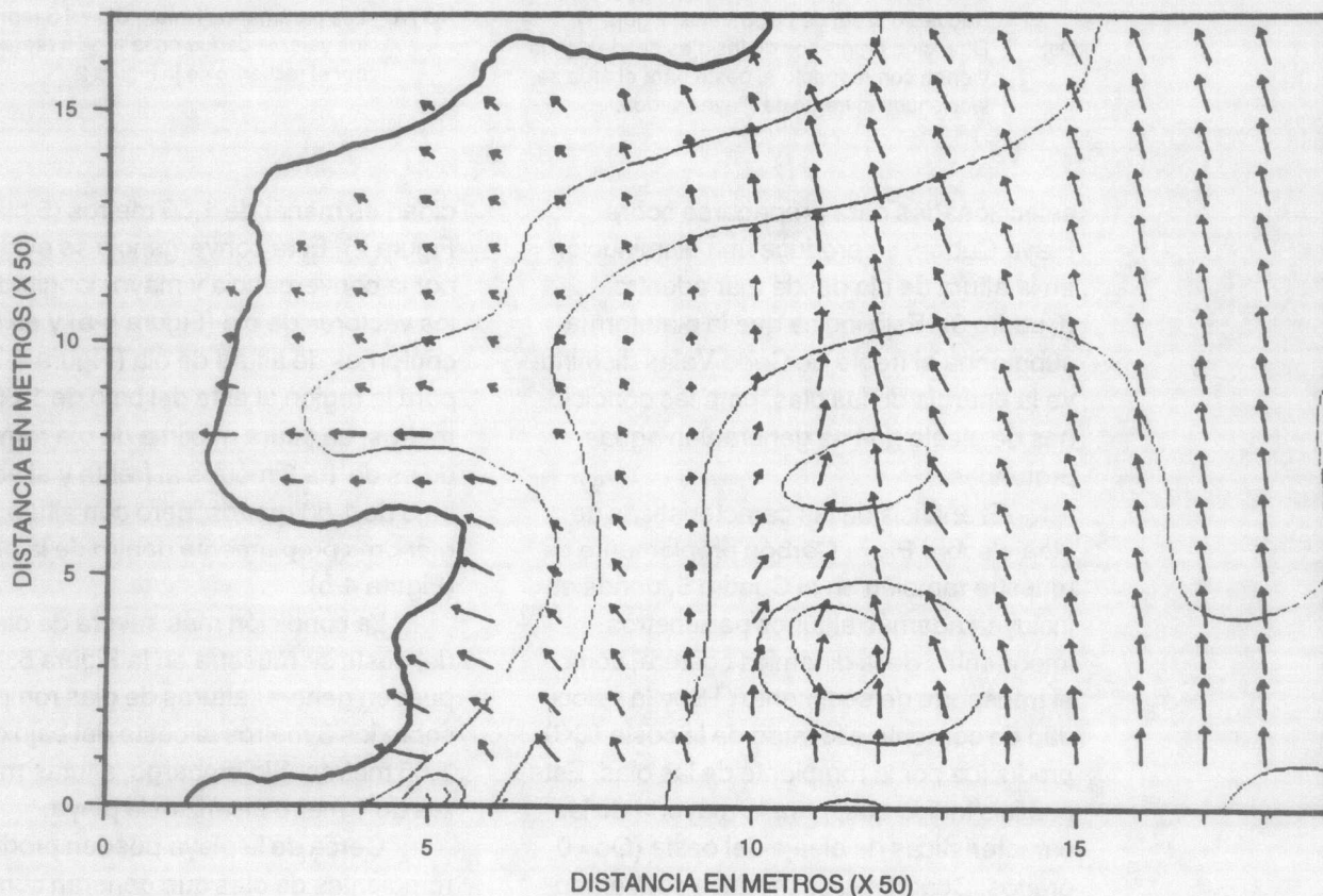
FIGURA 4-a. Vectores de ola en Playa Carbón, provincia de Guanacaste, para H_s=1,0 m, T=4,5 s y O_s=5,0 grad. (Abreviaciones en Cuadro 5).
