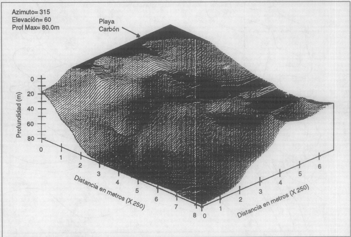
FIGURA 3. Batimetría en tres dimensiones de Playa Carbón, al sur de Cabo Velas, provincia de Guanacaste.
