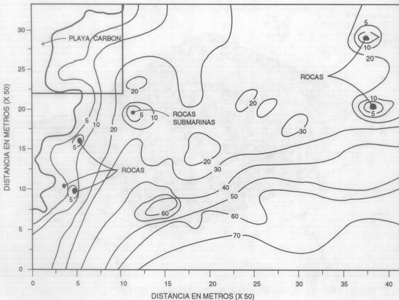
FIGURA 2. Contornos batimétricos de Playa Carbón al sur de Cabo Velas, provincia de Guanacaste.
