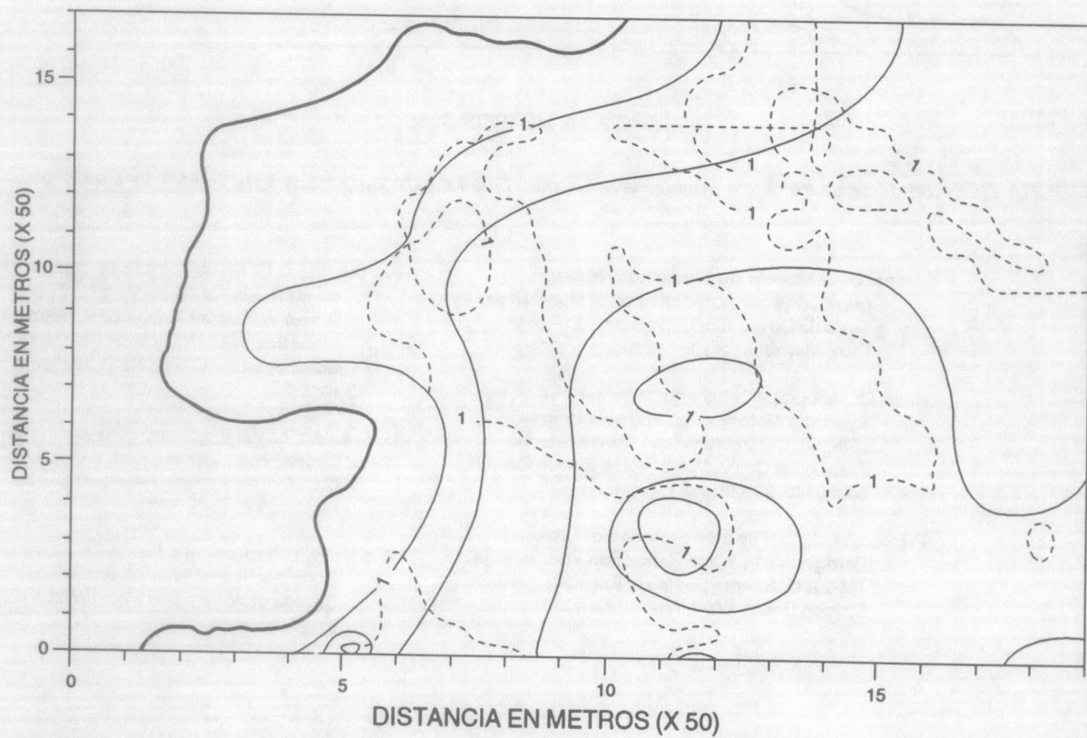
FIGURA 6-b. Contornos de altura de ola (m) en Playa Carbón, Guanacaste, para H_s=1,2 m, T=4,5 s y O_s=5,2 grd.
