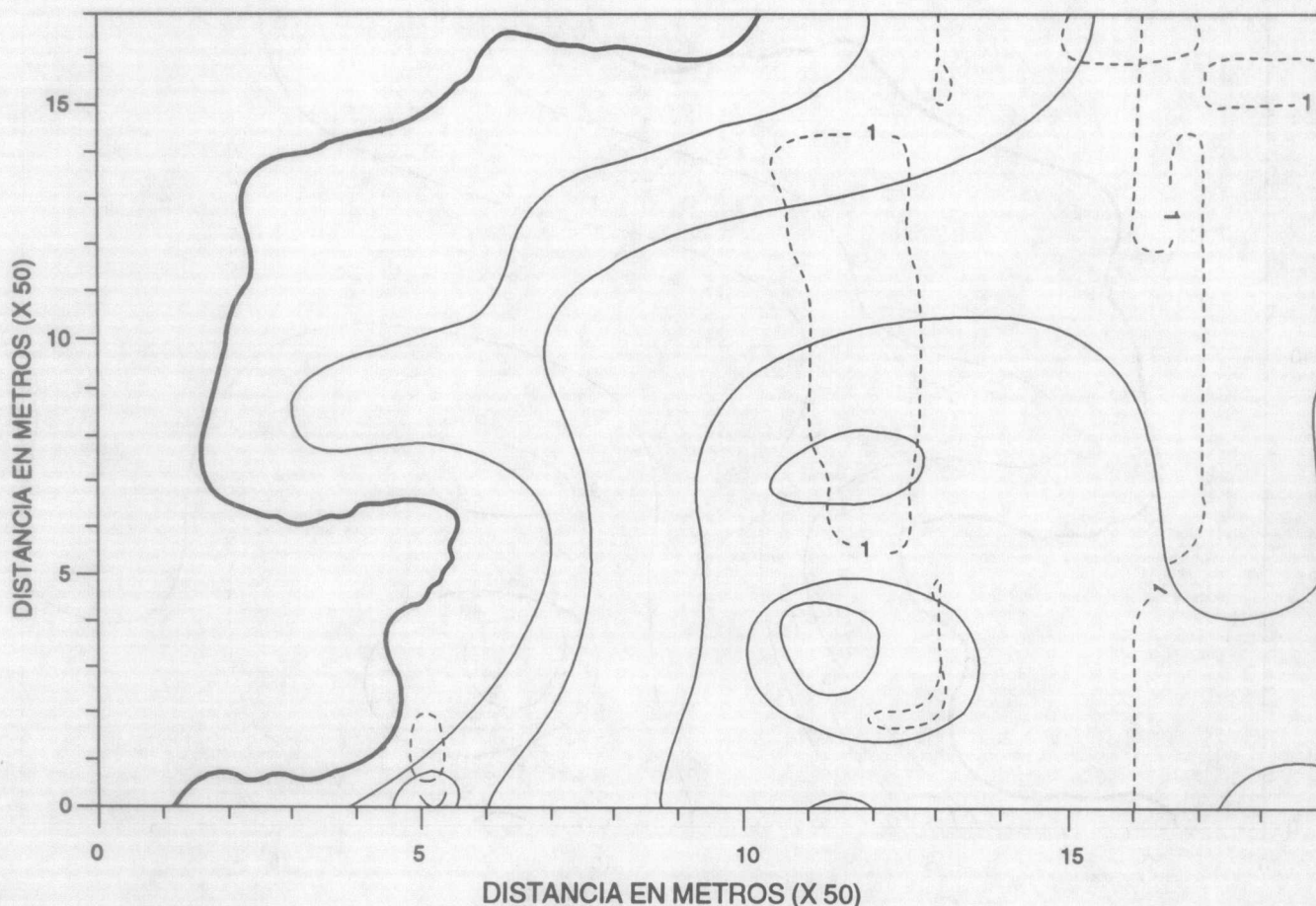
FIGURA 4-b. Contornos de altura de ola (m) en Playa Carbón, Guanacaste, para H_s=1,0 m, T=4,5 s y O_s=5,0 grd.
