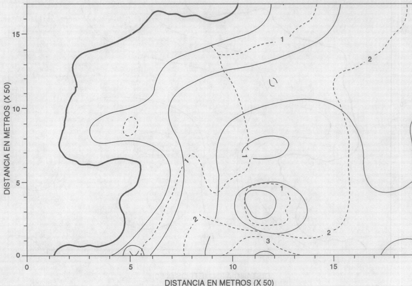
FIGURA 5. Contornos de altura de ola (m) en Playa Carbón, Guanacaste, para H_s=5,5 m, T=14,5 s y O_s=6,5 grd.
