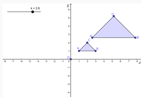
Figura 54: Homotecia del polígono ABC con un factor mayor que 1
