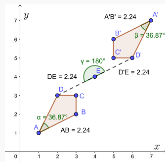
Figura 34: Medida del ángulo \angle DED'
