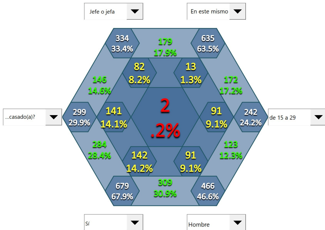
Figura 3: Correlación de unidades estadísticas en seis variables.
