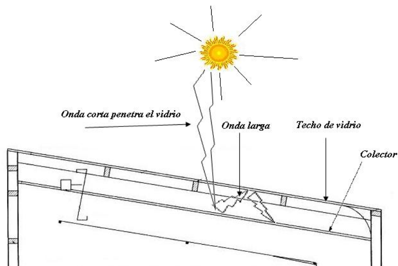
Figura 5. Efecto invernadero ocasionado por la incidencia de los rayos solares que atraviesan el techo de vidrio.
