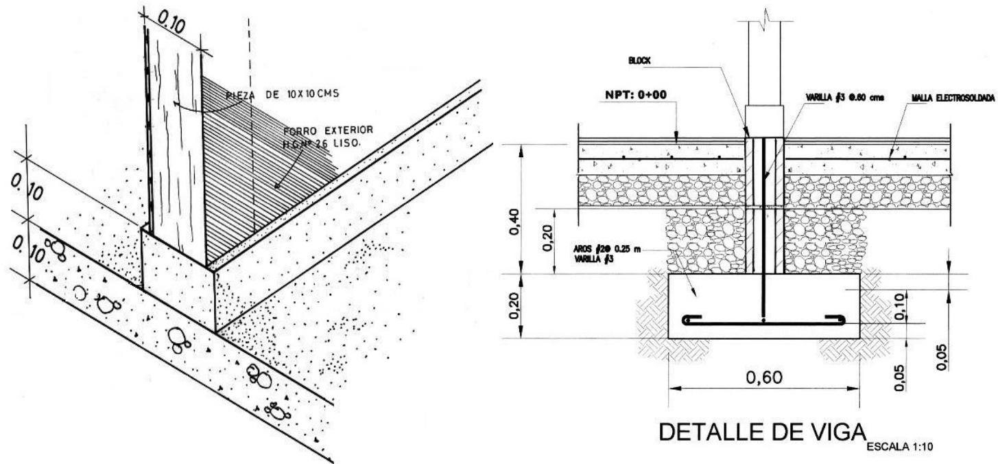
Detalle del cordón de concreto donde se monta la estructura de madera
